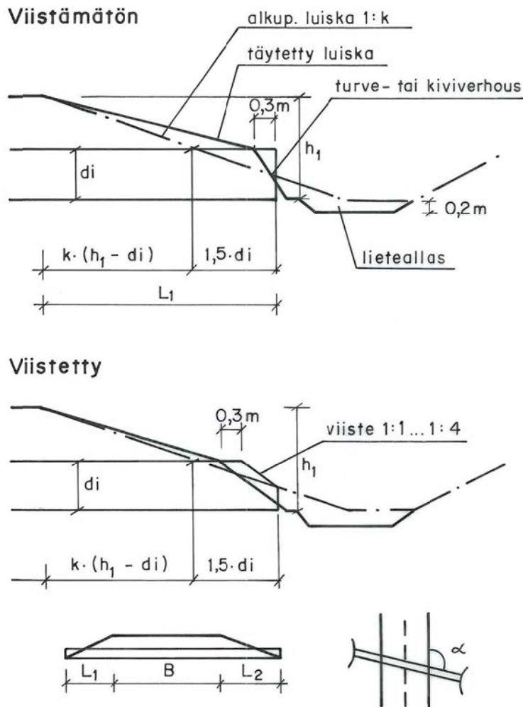
Kuva 25. Rummun pituuden määrittäminen.
