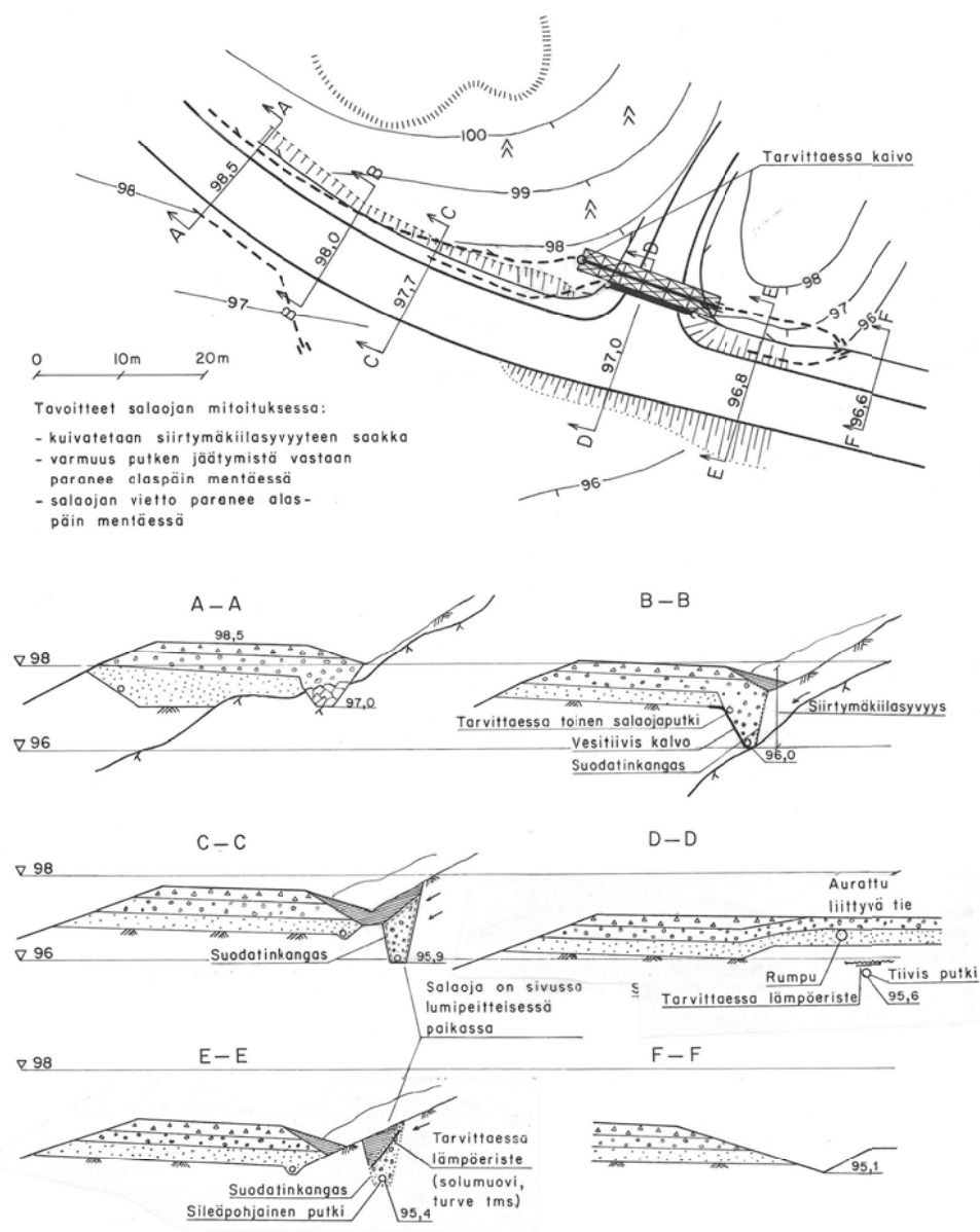
Kuva 29. Pohjavesivirtauksen katkaiseminen sivukaltevassa maastossa
