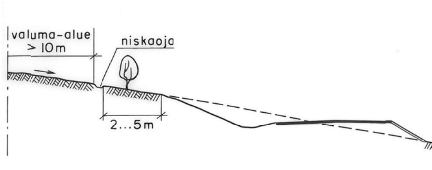
Kuva 19. Niskaojan sijainti maaleikkauksessa: niskaojat kaivetaan 0,2...0,5 m syviksi ja 0,4...0,8 leveiksi.
