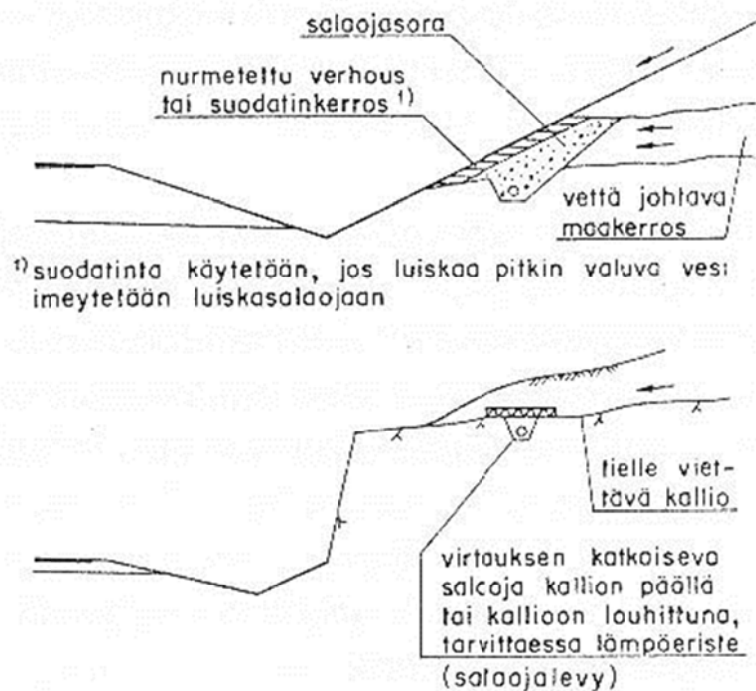
Kuva 30. Luiskasalaoja ja kallion päälle tehty niskasalaoja, joilla torjutaan paan-nejäättä tai luiskien syöpmistä.
