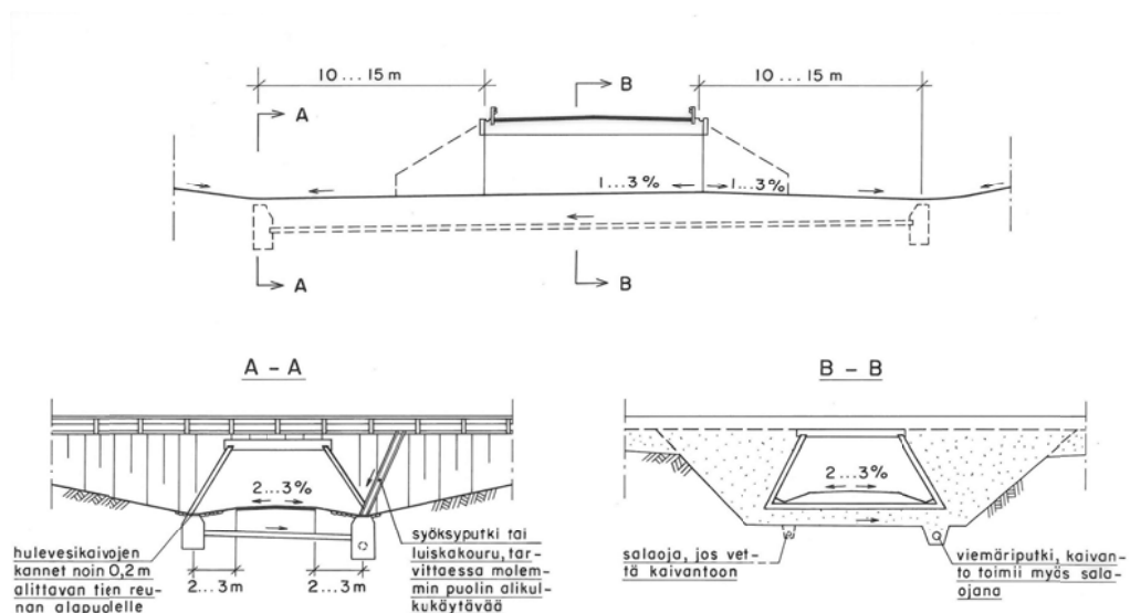
Kuva 15. Esimerkki alikulkukäytävän pintakuivatusjärjestelystä.
