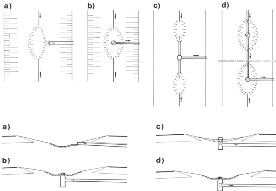
Kuva 10. Veden johtaminen keskialueelta: Leveältä ( > 10\text{ m} ) keskialueelta vesi poistetaan rummulla (a). Kapeammilta ( < 10\text{ m} ) keskialueilta vesi johdetaan kaivon (b) tai puolirummun (c) kautta.
