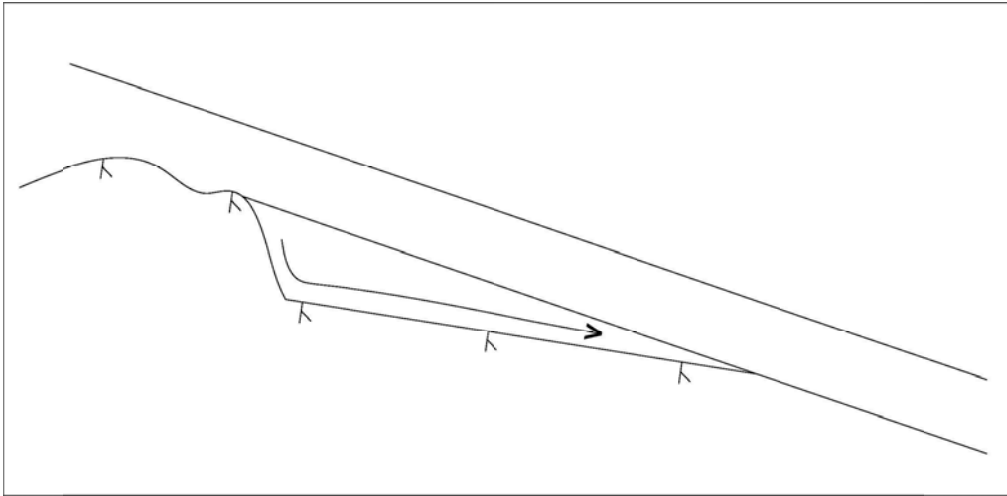
Kuva 28. Kallioleikkaukseen sijoitettavaa kiilaa kallistettaessa rakenteeseen suotautuva vesi ei jää taskuun vaan valuu pois rakenteesta.
