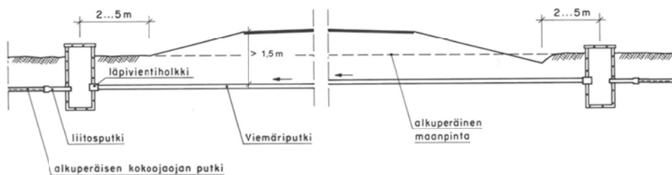
Kuva 32. Peltosalaojituksen kokoojaoja tien alituksessa. Tien ja sivuojien alapuolella salaojaputki korvataan halkaisijaltaan yhtä suurella viemäriputkella. Alempaa kaivoista ei tarvita, jos kokoojaojan purkuaukko on niin lähellä (<10 m) ja laskuputki niin suora, että mahdolliset tukokset voidaan poistaa tätä kautta. Routimattomalla pohjamaalla alempi kaivo tarvitaan vain pääteillä. Pehmeiköillä on varauduttava tien painumiseen.
