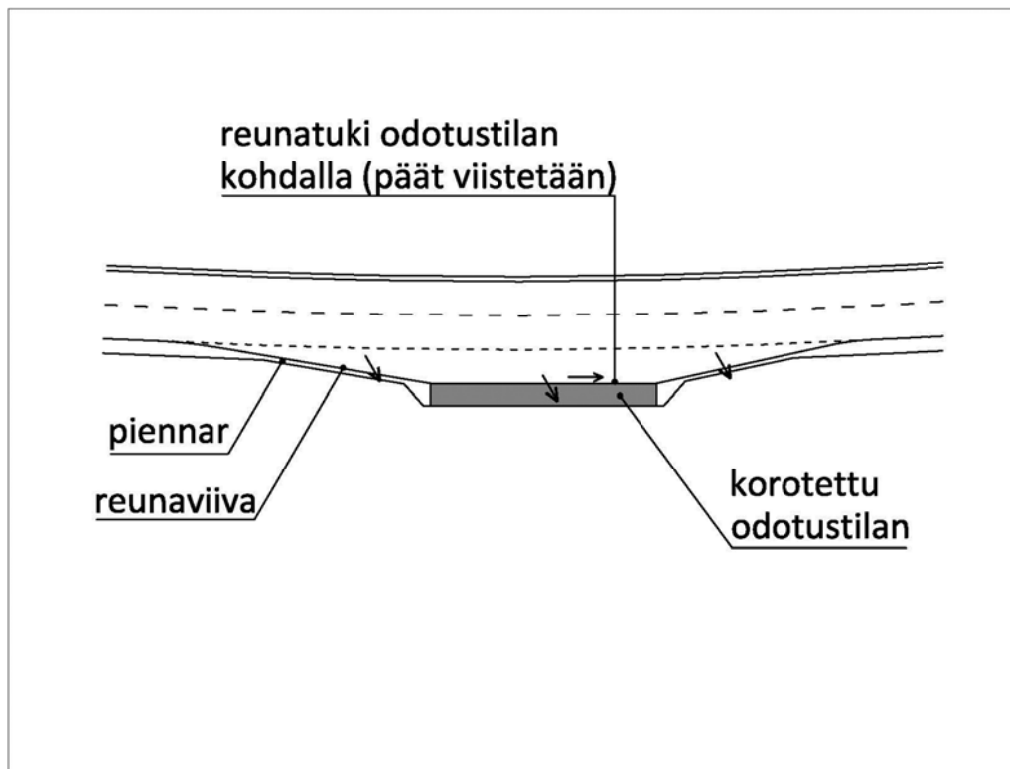
Kuva 13. Esimerkki korotetulla odotustilalla varustetun linja-autopysäkin pinta-kuivatuksesta. Nuolet osoittavat veden valumissuuntaa. Taajamassa reumatuki voi kiertää koko pysäkkitaskun.
