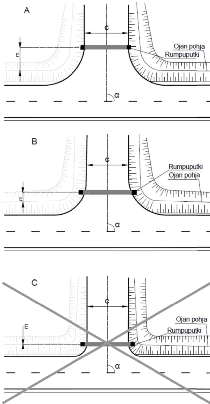
Kuva 24. Liittymärummun sijoittaminen. Sivuojarummun sijoituksesta on kerrottu tarkemmin ohjeessa
